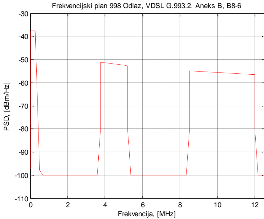
Slika 5.6.2 Frekvencijski predložak za odlazni smjer prijensa za VDSL2, frekvencijski plan 998, B8-6
